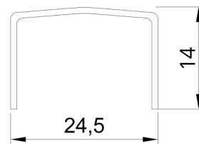
Corte Transversal Perfil
