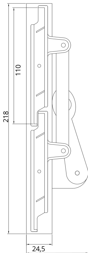
Mecanismo Cerrado
