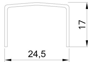
Corte Transversal Perfil
