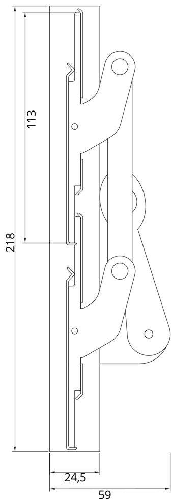
Mecanismo Cerrado
