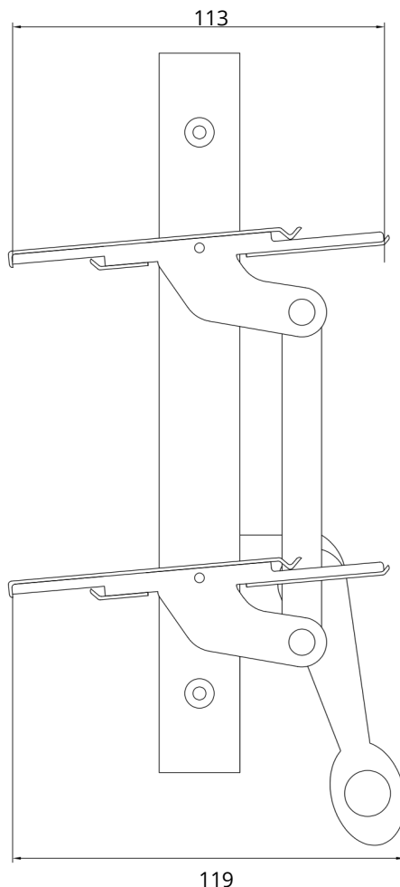
Mecanismo Abierto
